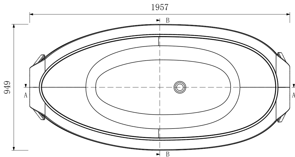
俯视图
