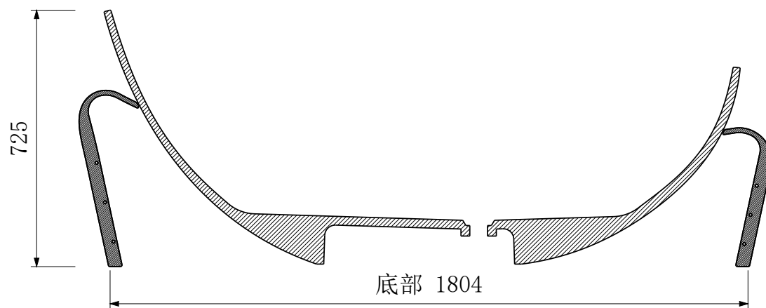
A-A 纵向中心剖面
