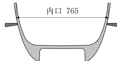
B-B 横向中心剖面
