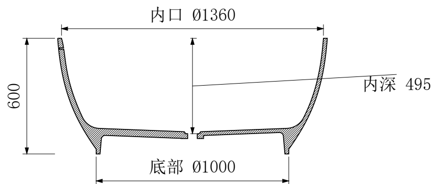
A-A 中心剖面
