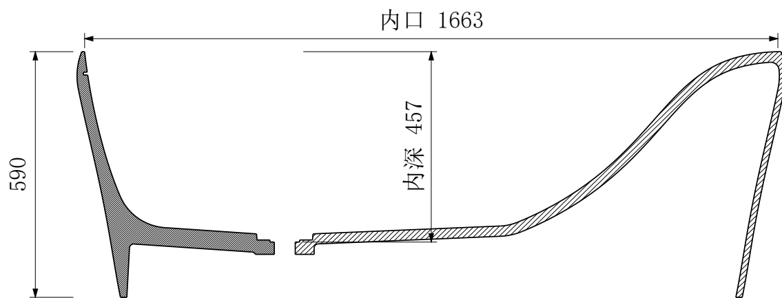
A-A 纵向中心剖面
