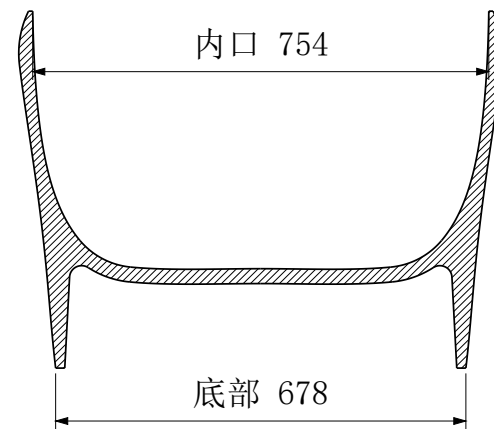
B-B 横向中心剖面
