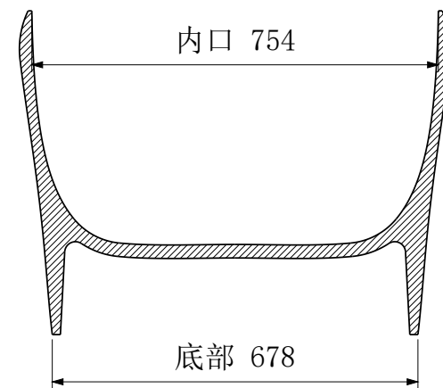
B-B 横向中心剖面
