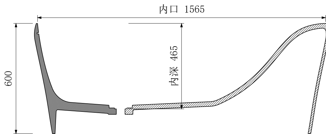
A-A 纵向中心剖面
