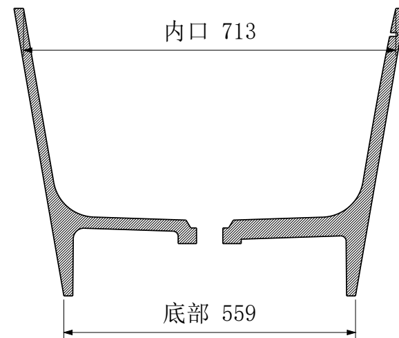
B-B 横向中心剖面
