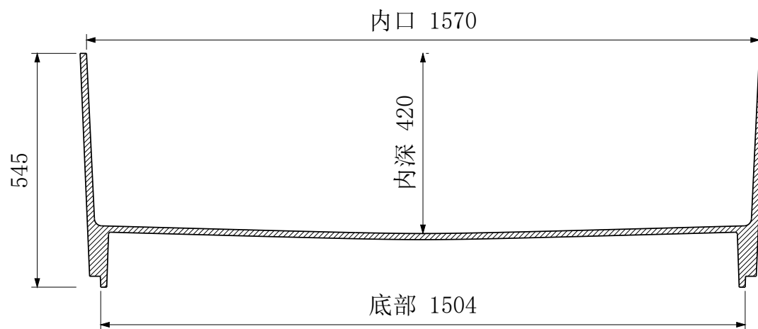
A-A 纵向中心剖面
