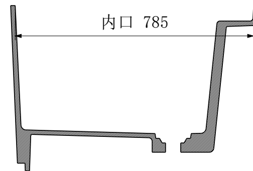
B-B 横向中心剖面
