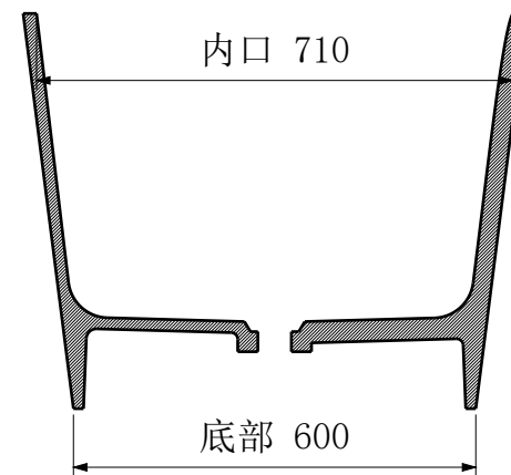
B-B 横向中心剖面
