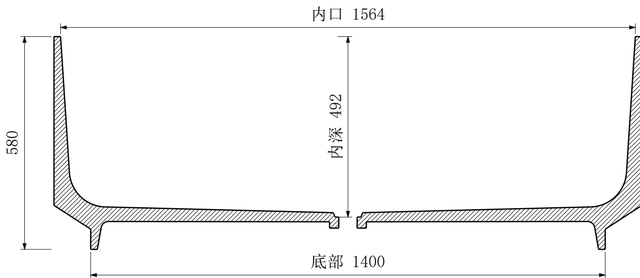
A-A 纵向中心剖面
