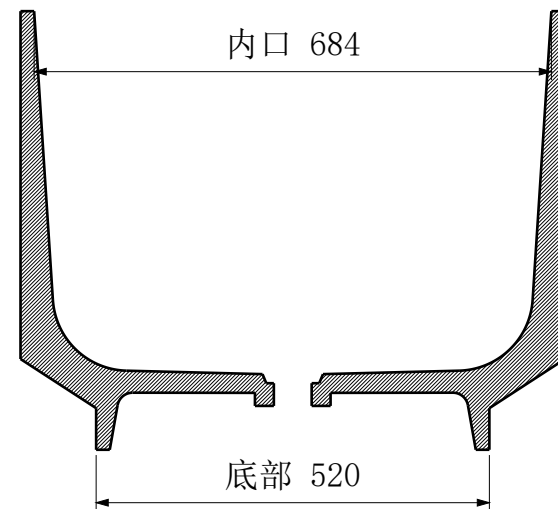
B-B 横向中心剖面
