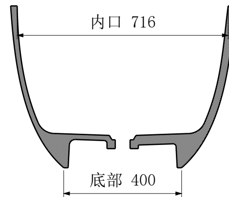
B-B 横向中心剖面
