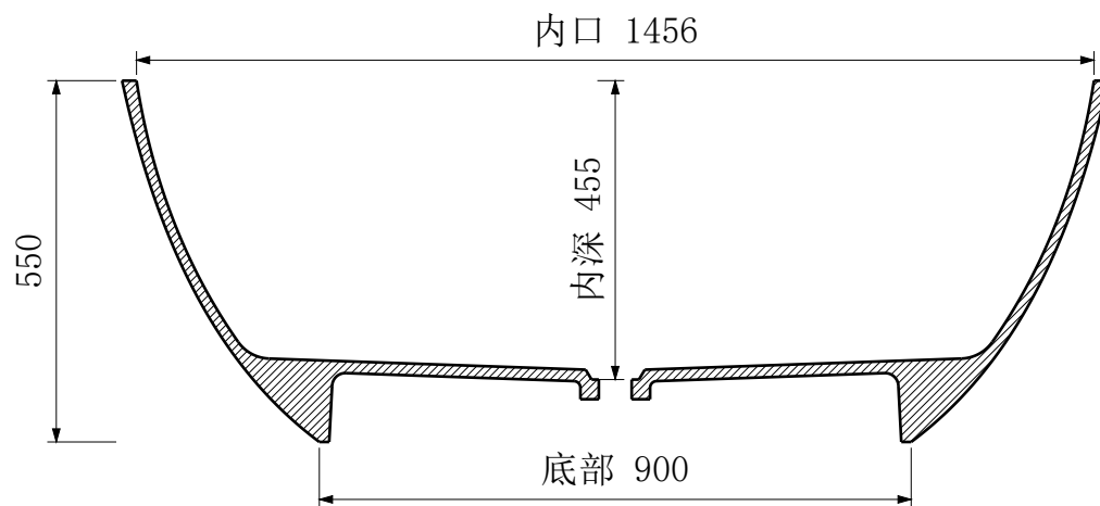
A-A 纵向中心剖面
