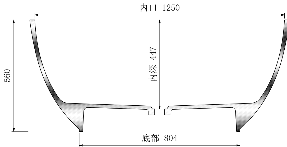
A-A 纵向中心剖面
