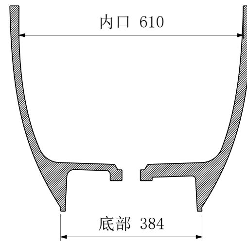
B-B 横向中心剖面
