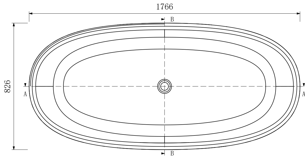
俯视图
