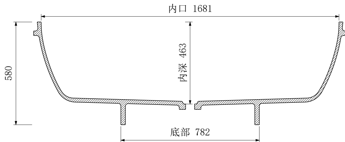
A-A 纵向中心剖面
