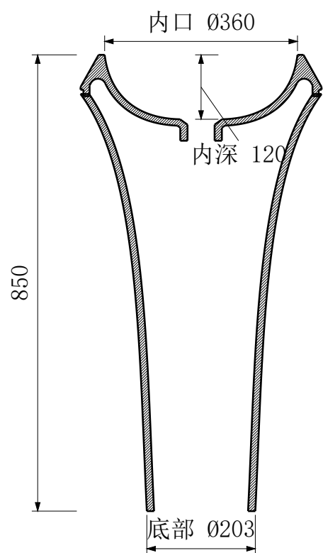
A-A 中心剖面
