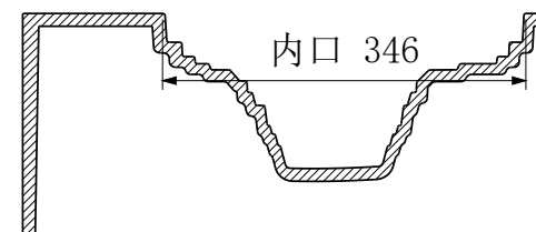
B-B 横向中心剖面
