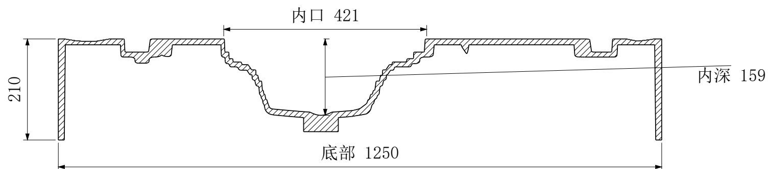
A-A 纵向中心剖面
