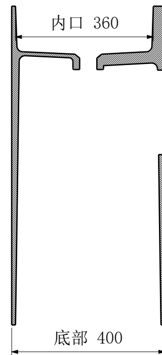
B-B 横向中心剖面
