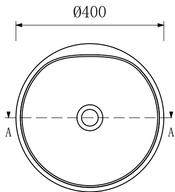
俯视图
