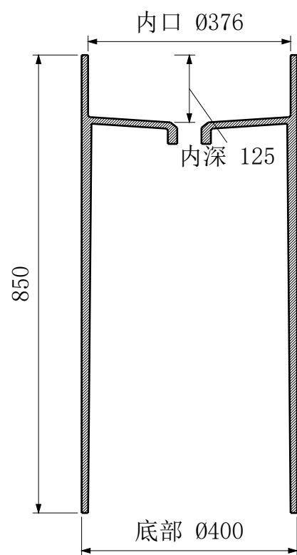
A-A 中心剖面
