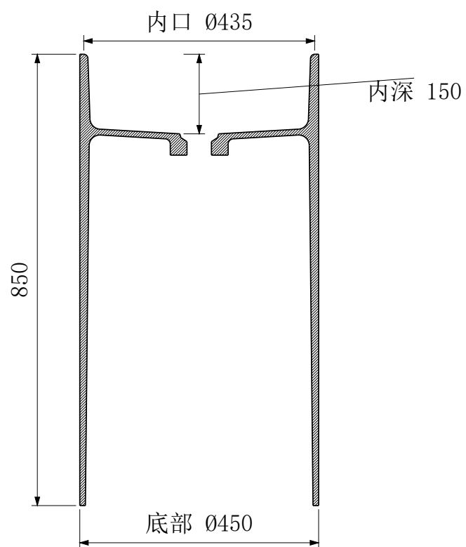
A-A 中心剖面
