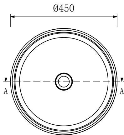
俯视图
