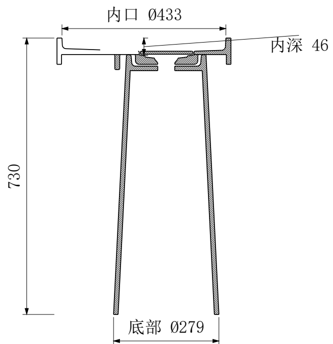
A-A 中心剖面
