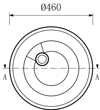
俯视图
