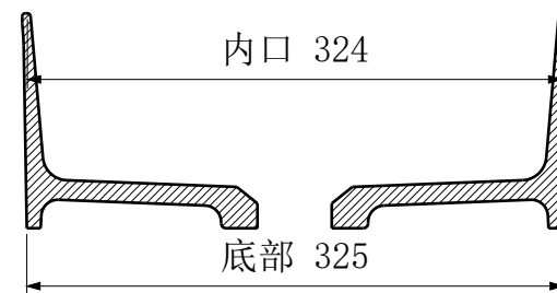
B-B 横向中心剖面
