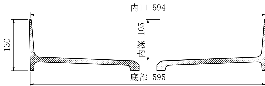
A-A 纵向中心剖面
