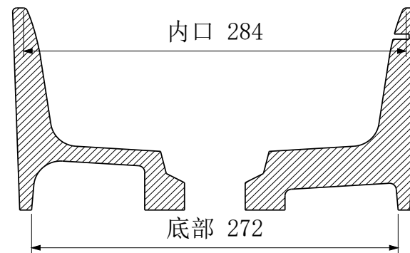
B-B 横向中心剖面
