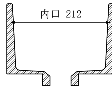
B-B 横向中心剖面
