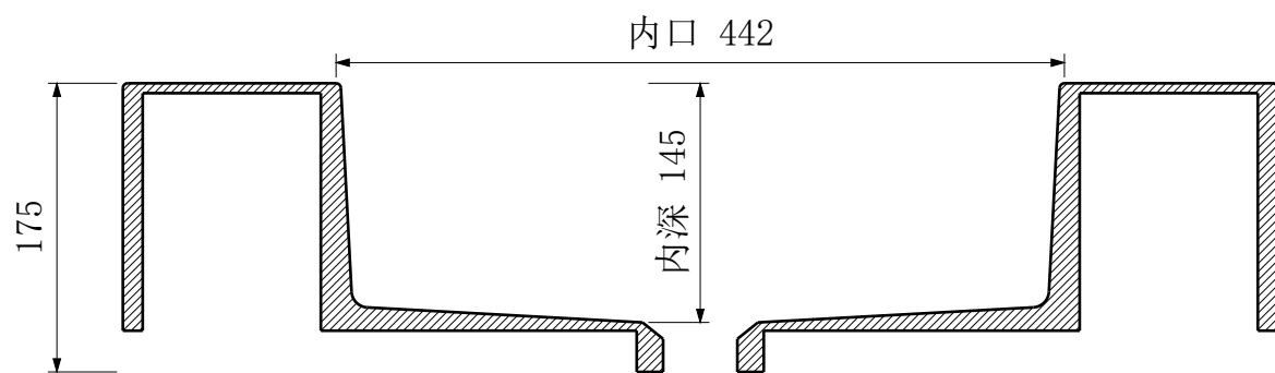
A-A 纵向中心剖面
