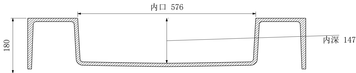
A-A 纵向中心剖面
