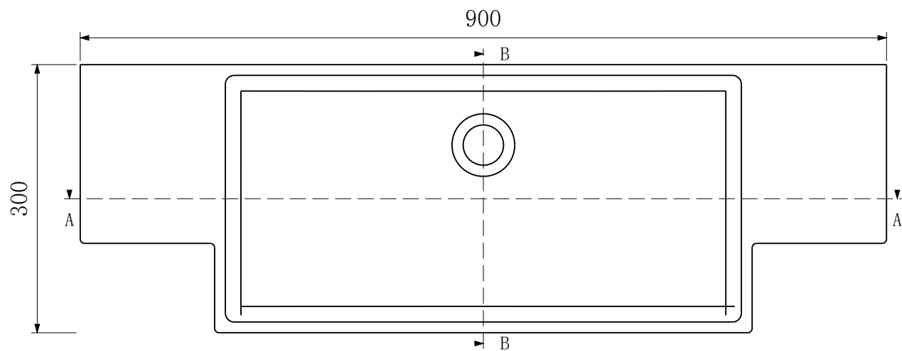
俯视图
