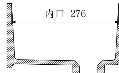
B-B 横向中心剖面
