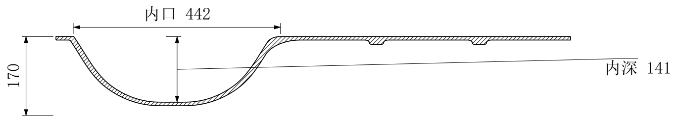
A-A 纵向中心剖面
