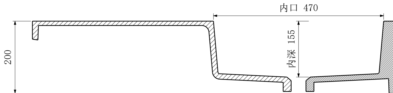
A-A 纵向中心剖面
