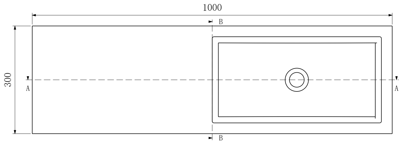
俯视图
