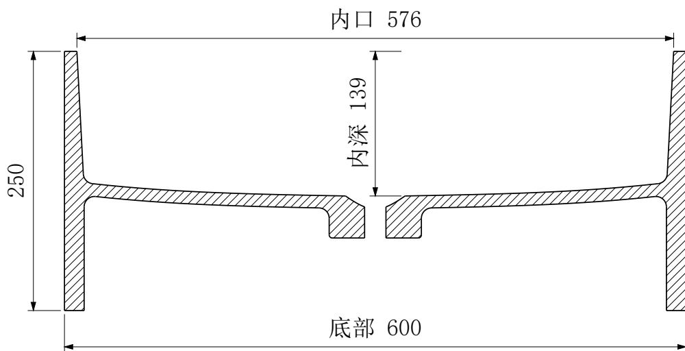
A-A 纵向中心剖面
