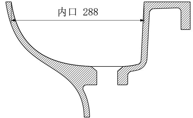
B-B 横向中心剖面
