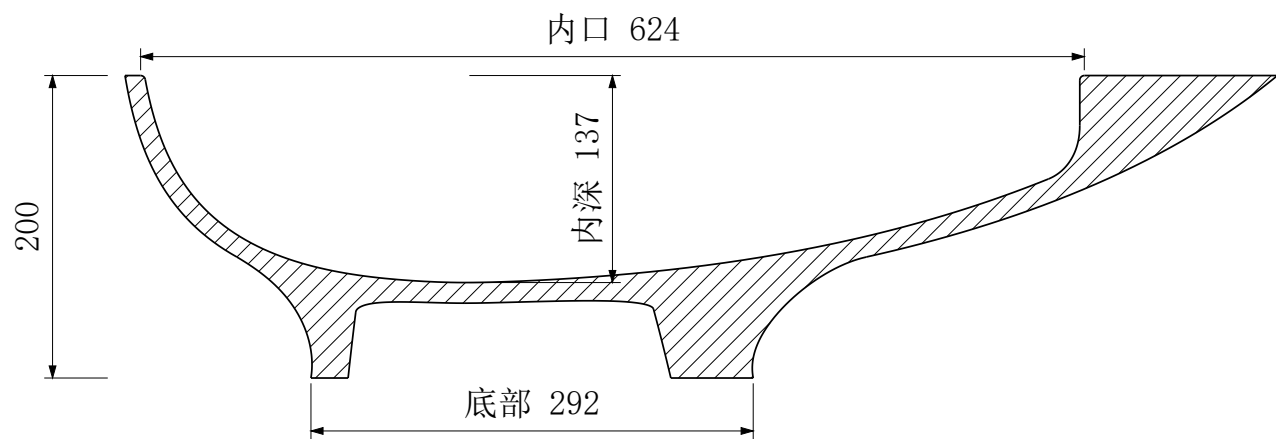
A-A 纵向中心剖面
