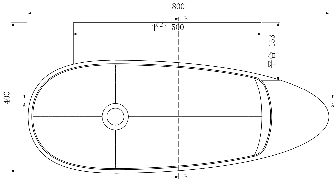
俯视图
