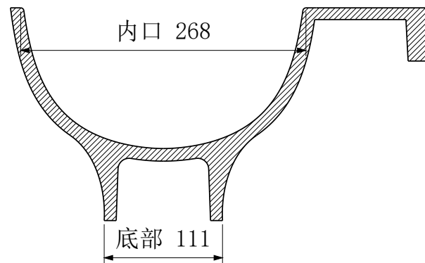
B-B 横向中心剖面
