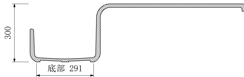
A-A 纵向中心剖面
