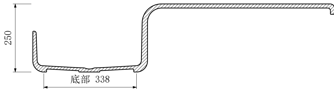
A-A 纵向中心剖面
