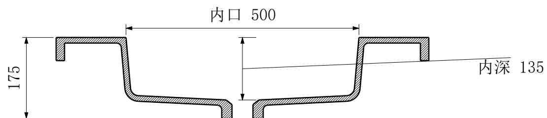
A-A 纵向中心剖面
