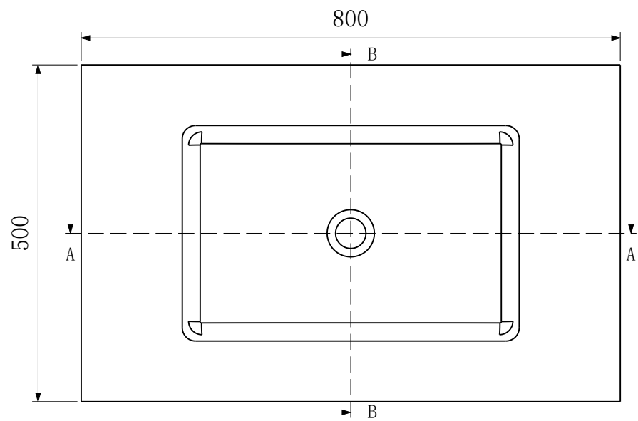
俯视图
