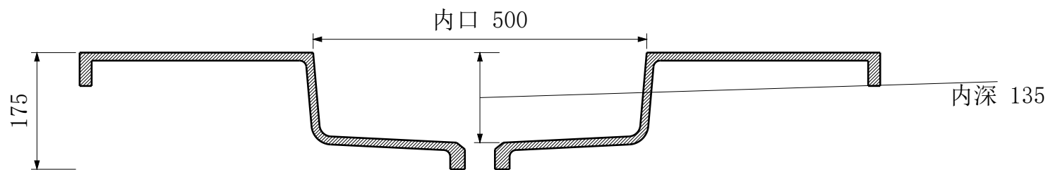
A-A 纵向中心剖面
