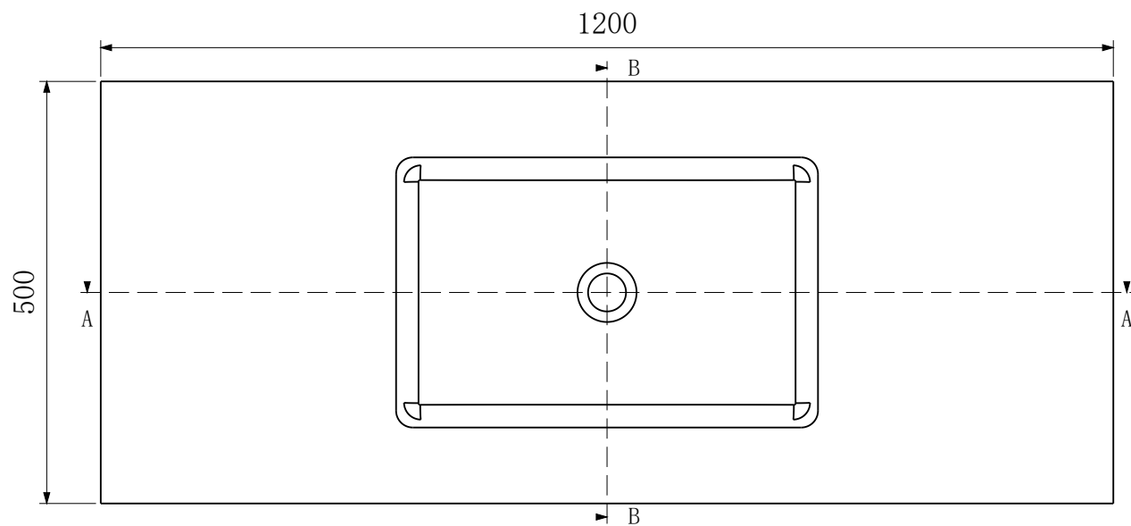
俯视图
