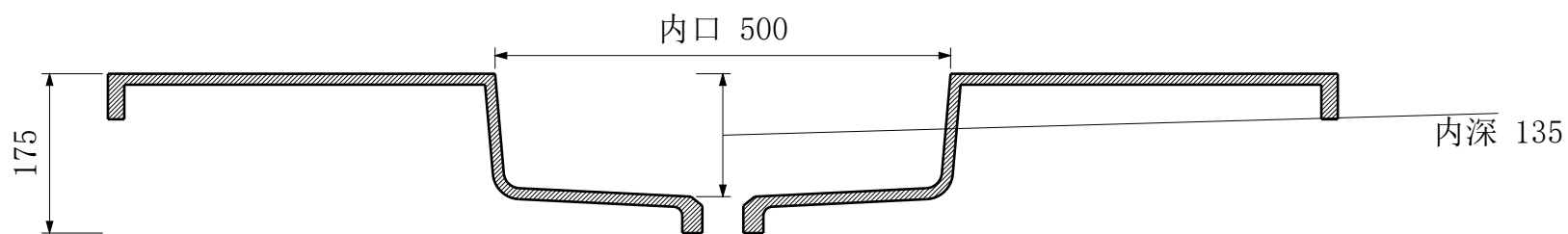
A-A 纵向中心剖面
