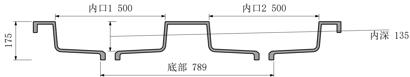
A-A 纵向中心剖面
