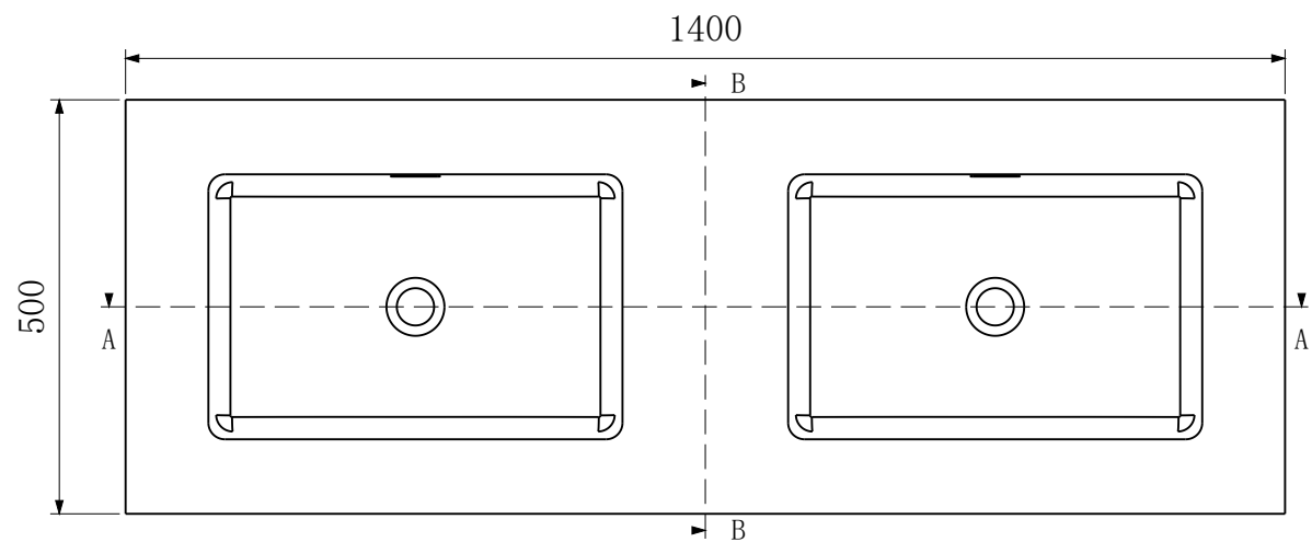
俯视图
