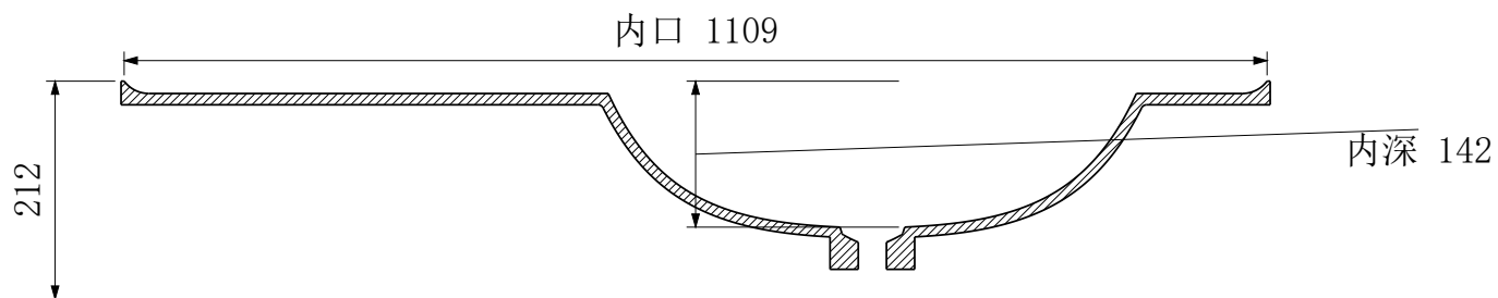
A-A 纵向中心剖面
