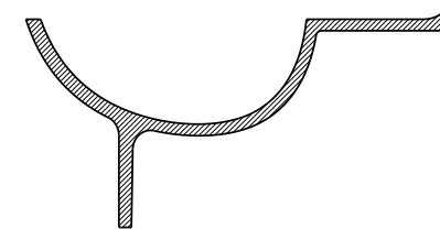
B-B 横向中心剖面
