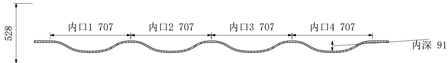
A-A 纵向中心剖面
