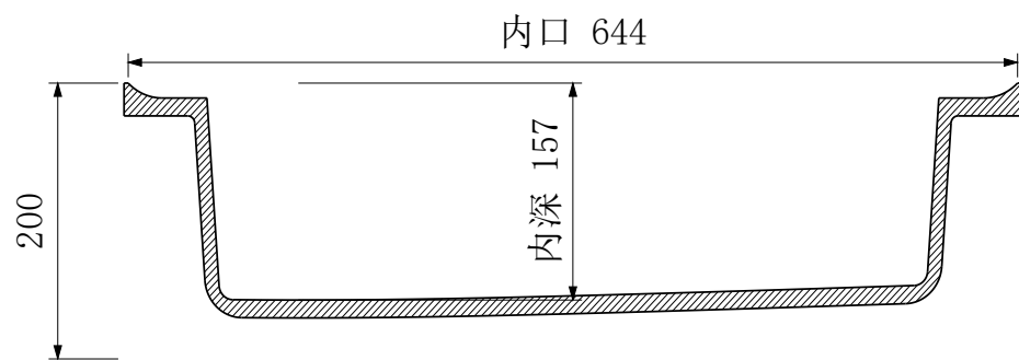
A-A 纵向中心剖面
