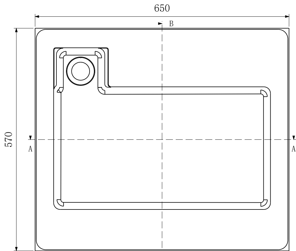
俯视图
