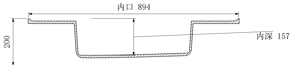
A-A 纵向中心剖面
