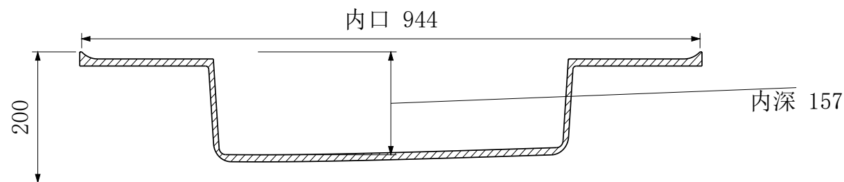
A-A 纵向中心剖面
