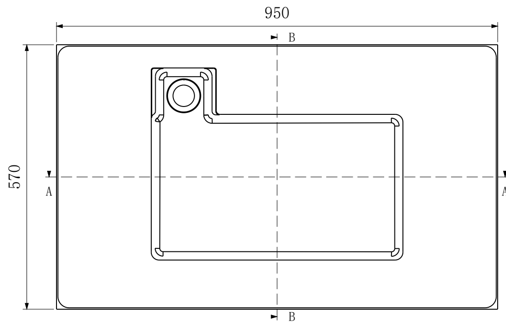
俯视图
