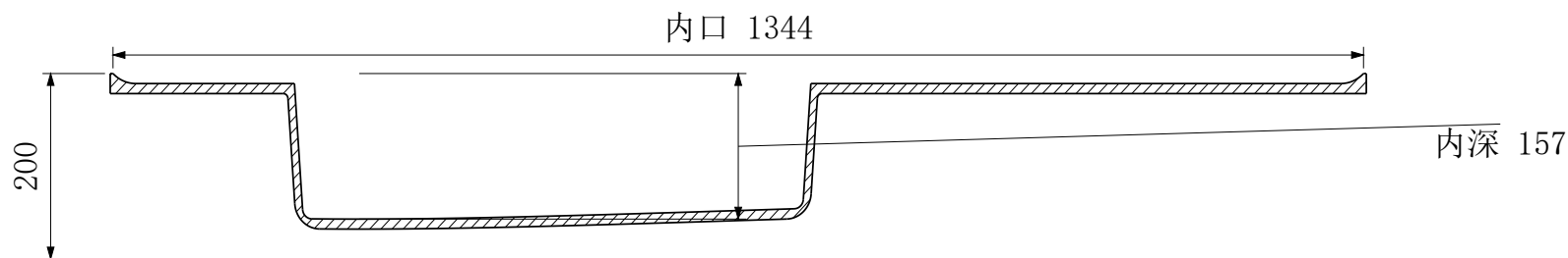
A-A 纵向中心剖面
