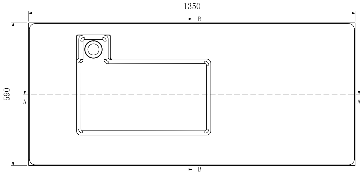
俯视图
