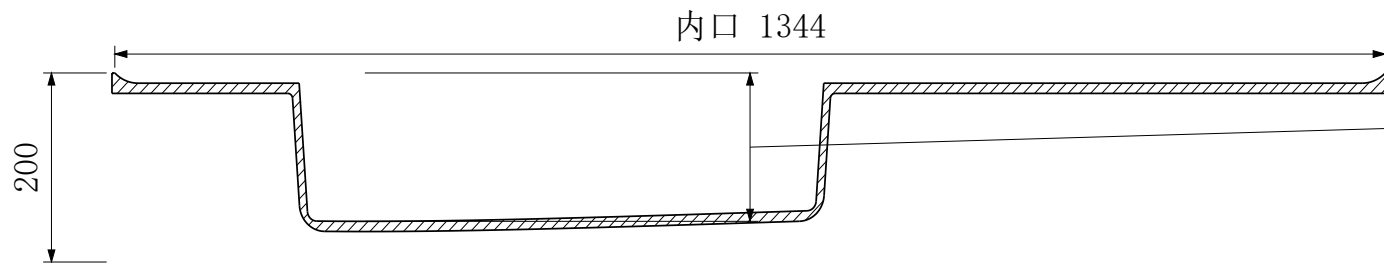
A-A 纵向中心剖面
