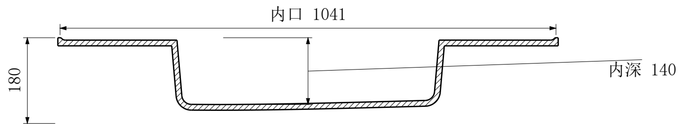
A-A 纵向中心剖面
