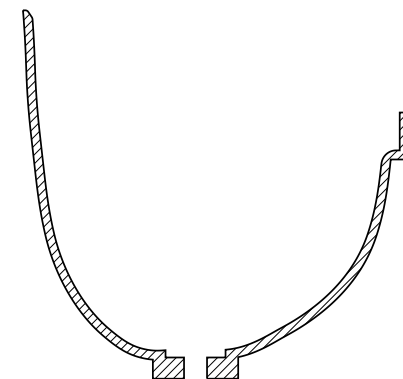
B-B 横向中心剖面
