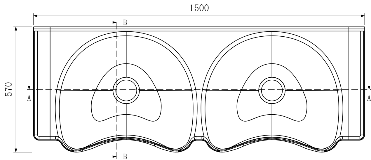
俯视图
