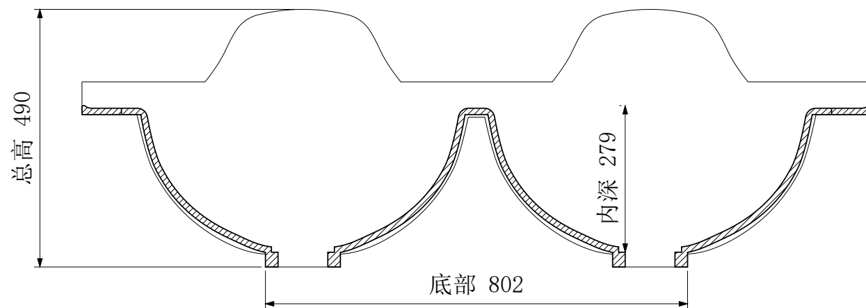
A-A 纵向中心剖面
