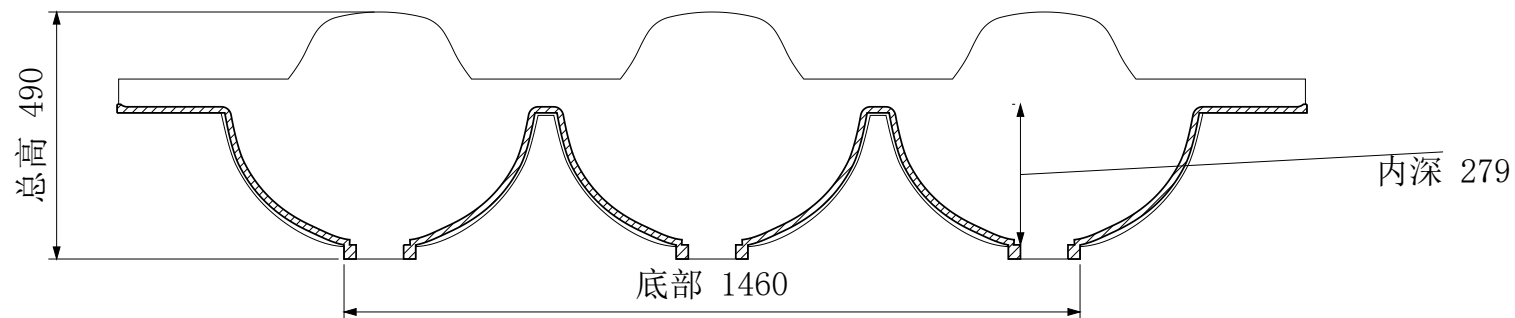
A-A 纵向中心剖面
