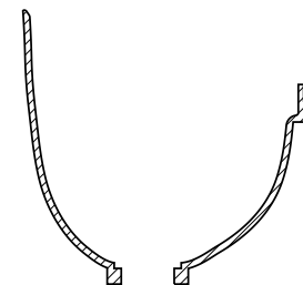
B-B 横向中心剖面
