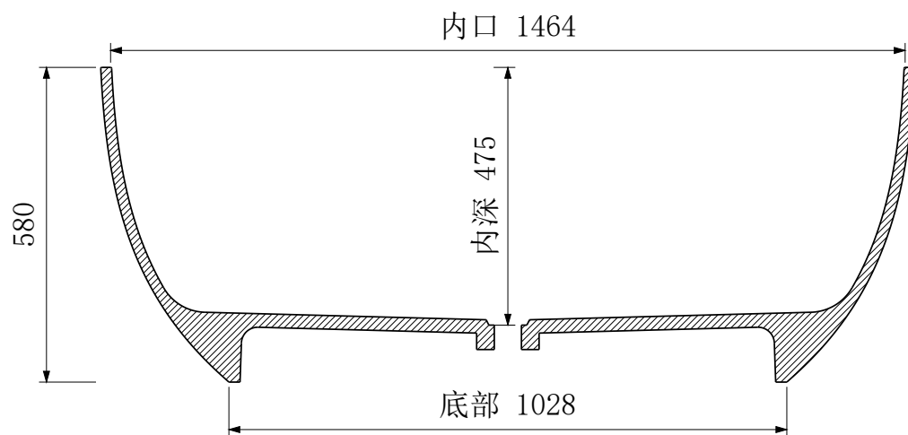
A-A 纵向中心剖面
