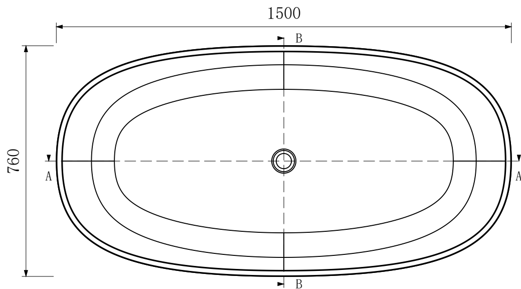
俯视图
