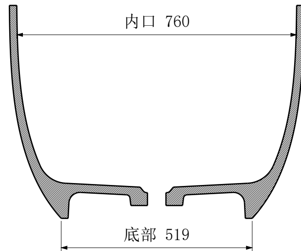
B-B 横向中心剖面
