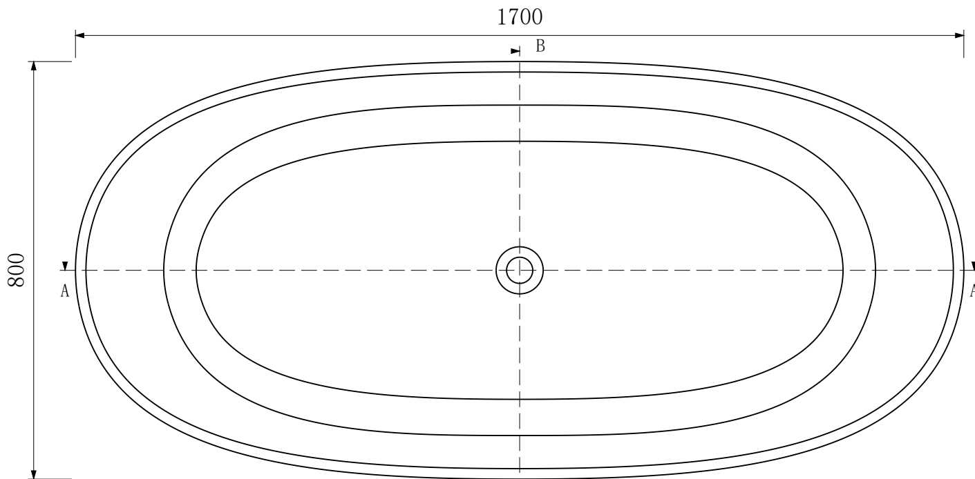
俯视图
