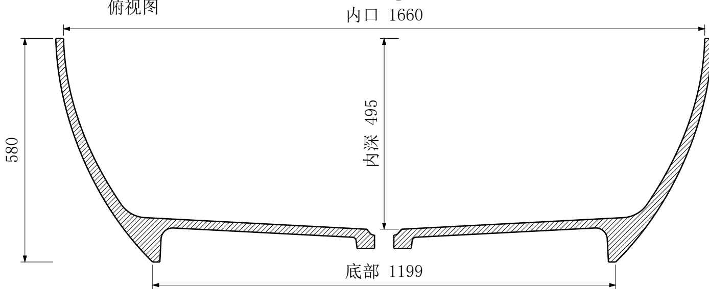
A-A 纵向中心剖面
