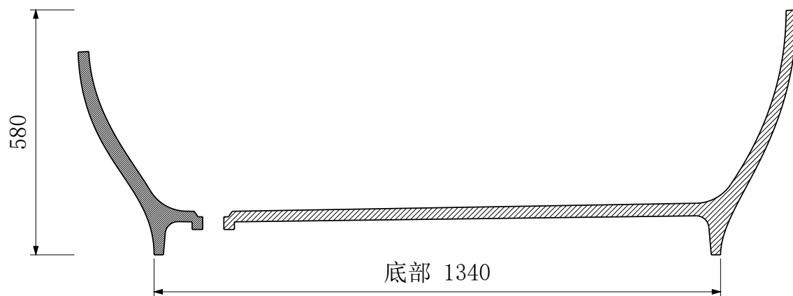
A-A 纵向中心剖面
