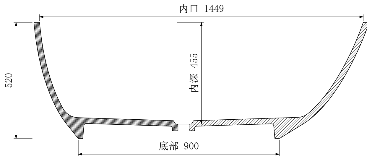
A-A 纵向中心剖面
