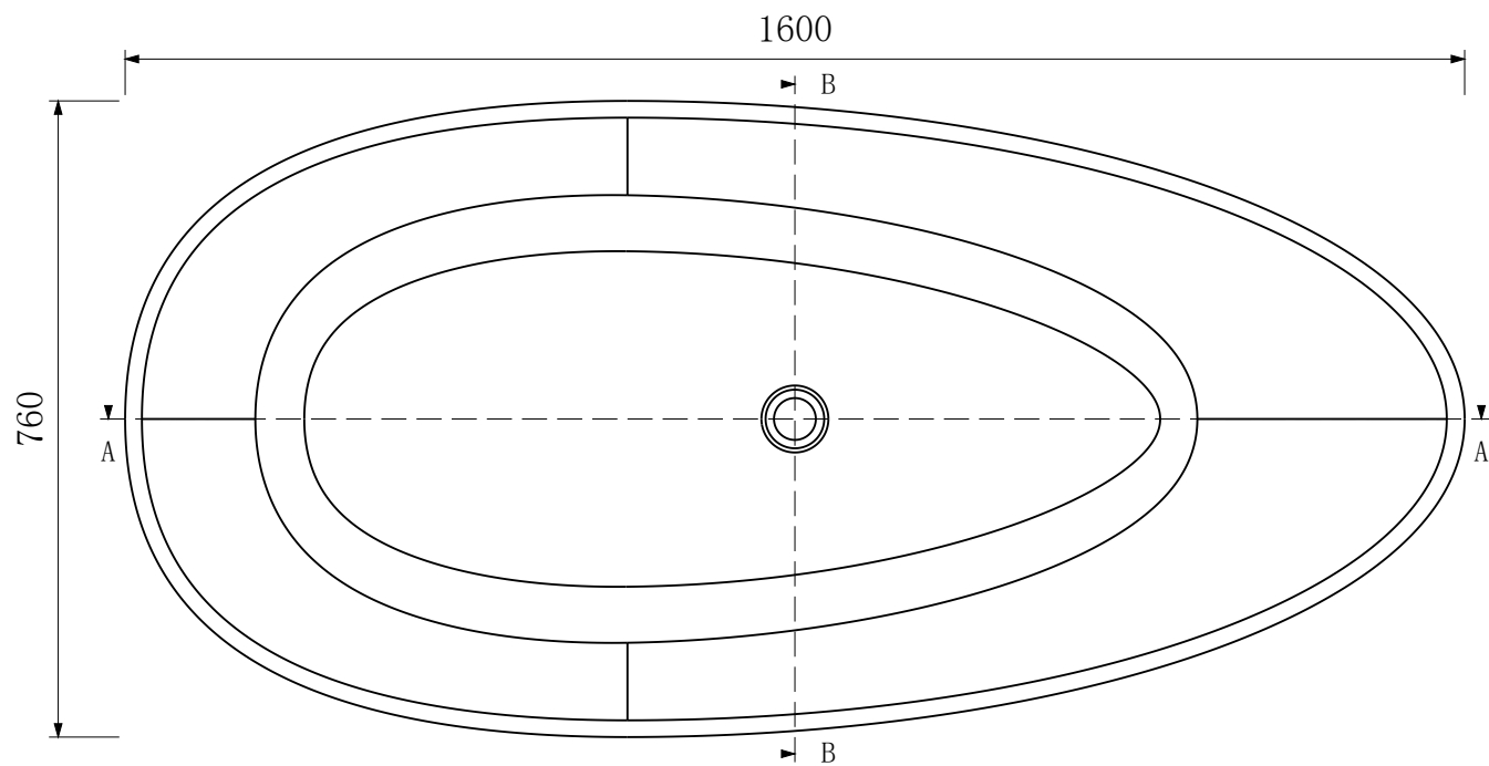
俯视图
