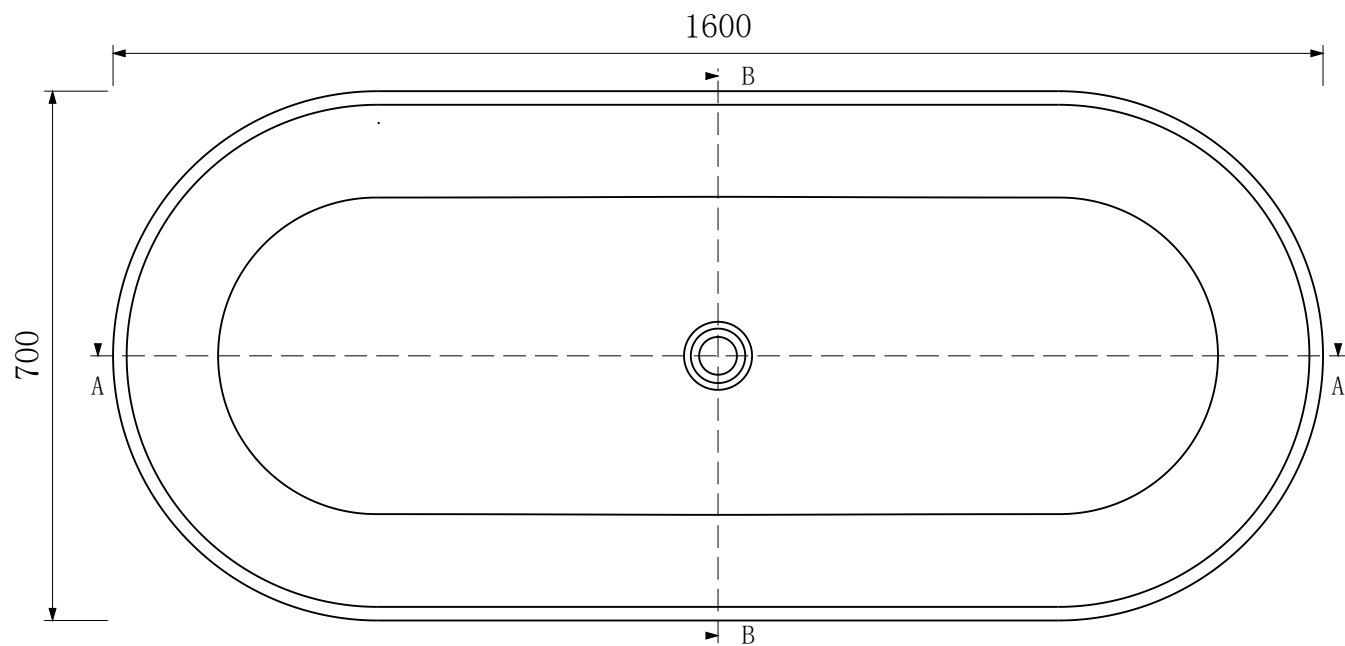
俯视图
