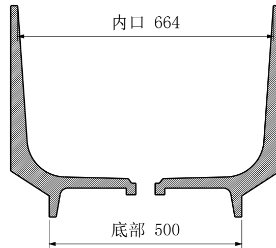
B-B 横向中心剖面
