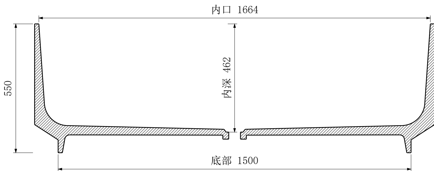
A-A 纵向中心剖面
