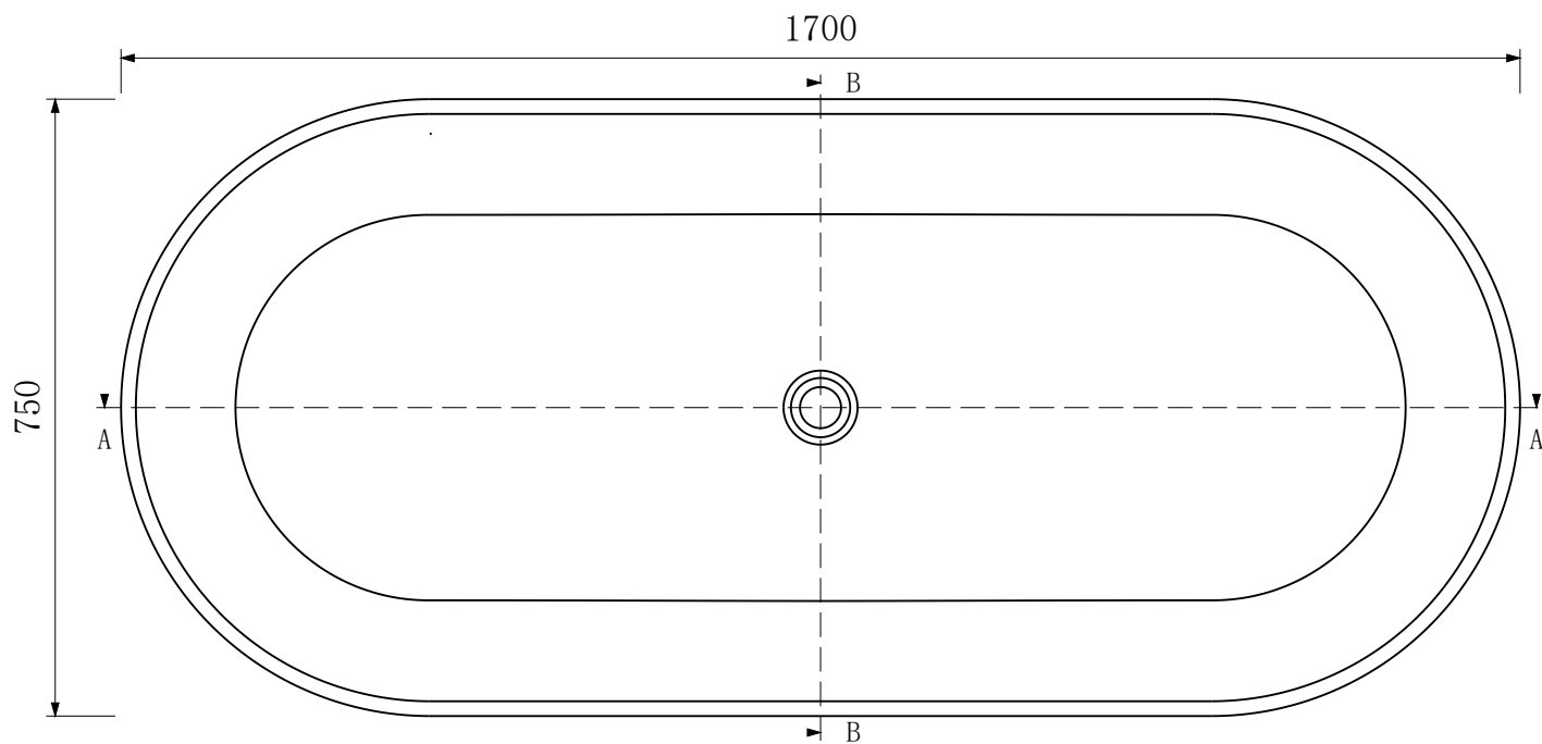
俯视图
